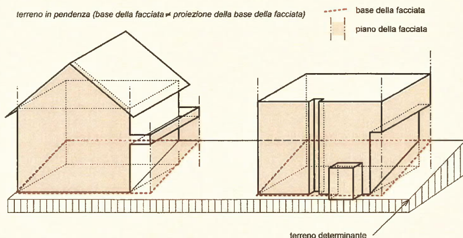
Figure 3.1 – 3.3 Piano della facciata e base delle facciate
