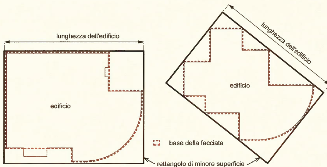
Figura 4.1 Lunghezza dell'edificio
