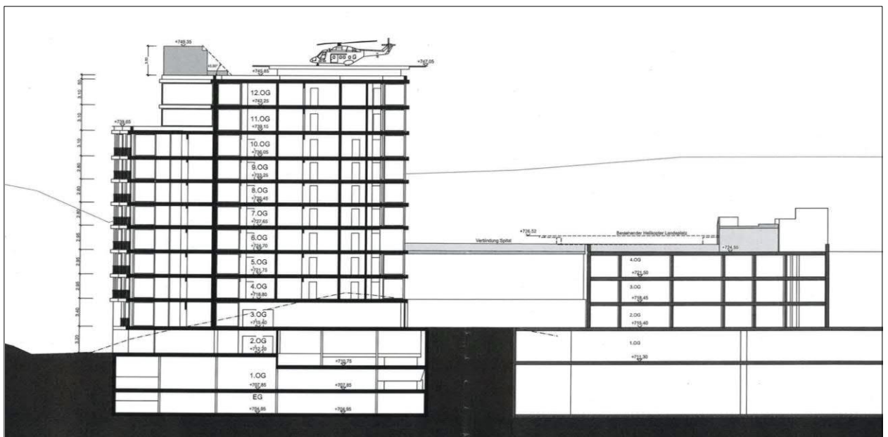
Schnitt Alters- und Gesundheitsresidenz / Regionalspital Ilanz mit Helikopter-Landeplatz und Passerelle zum Regionalspital
