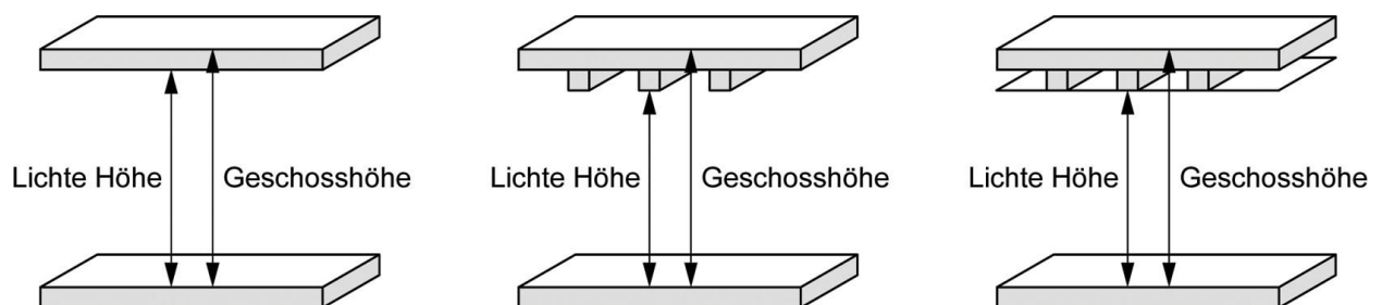
Figur 5.4 Lichte Höhe
