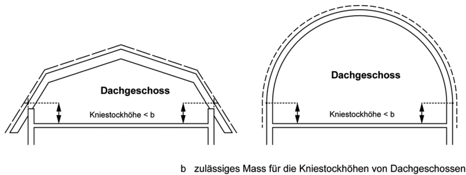
Figur 6.3 Dachgeschosse
