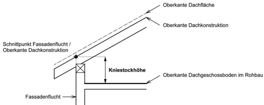
Figur 5.3 Kniestockhöhe
