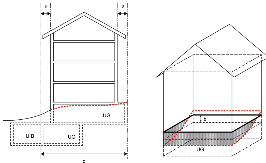
Figur 6.2 Untergeschosse
