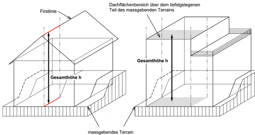
Figur 5.1 Gesamthöhe
