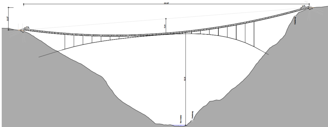
Abbildung 4: Längsschnitt aus technischem Bericht, Casutt Wyrsh Zwicky AG
