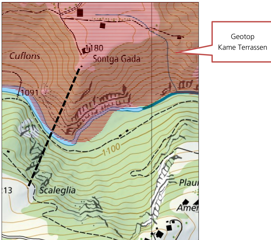
Abbildung 6: Ausschnitt Geotop Nr. 284 Kame Terrassen mit Linienführung der Hängebrücke
