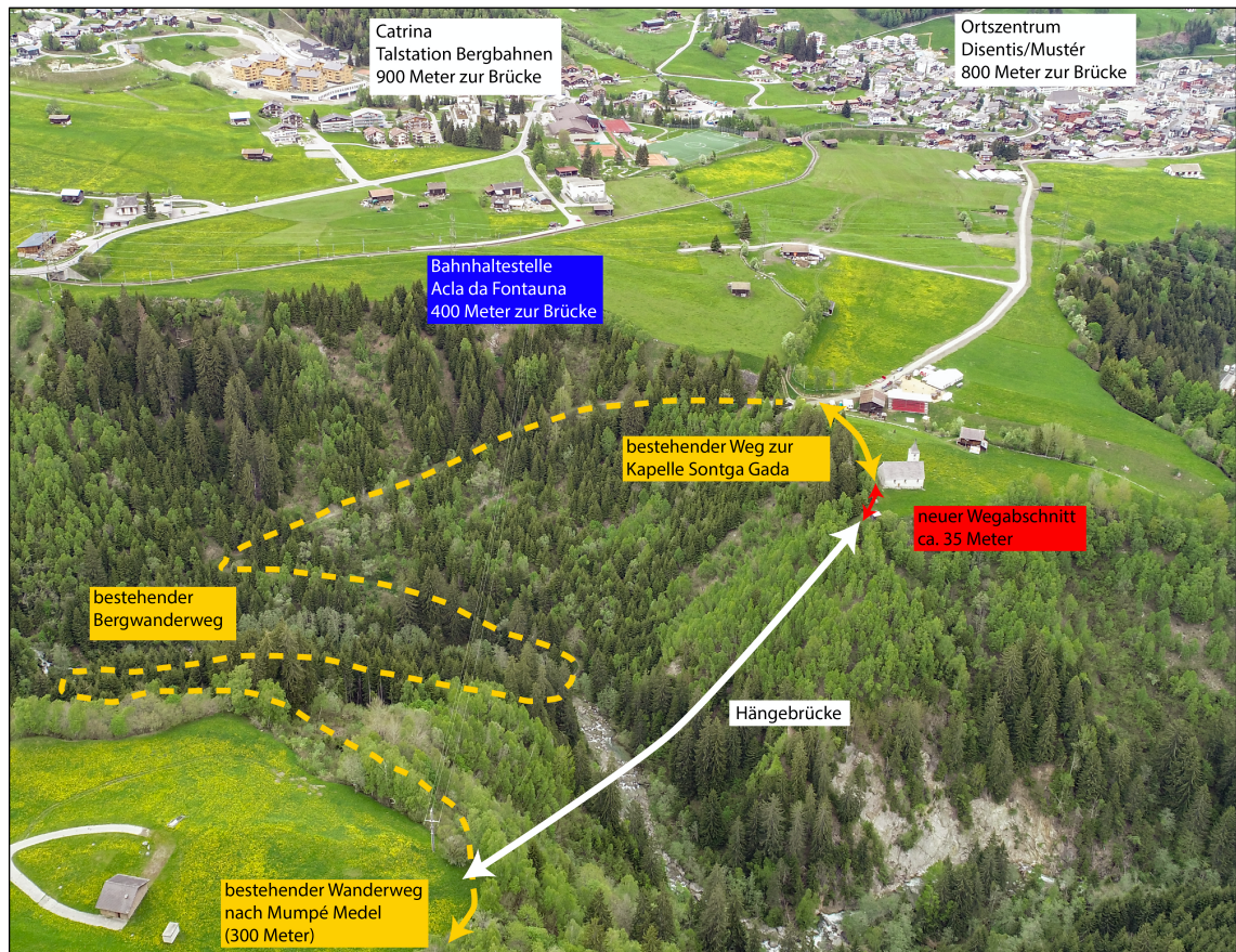
Abbildung 5: Ansicht Hängebrücke mit Wegverbindungen
