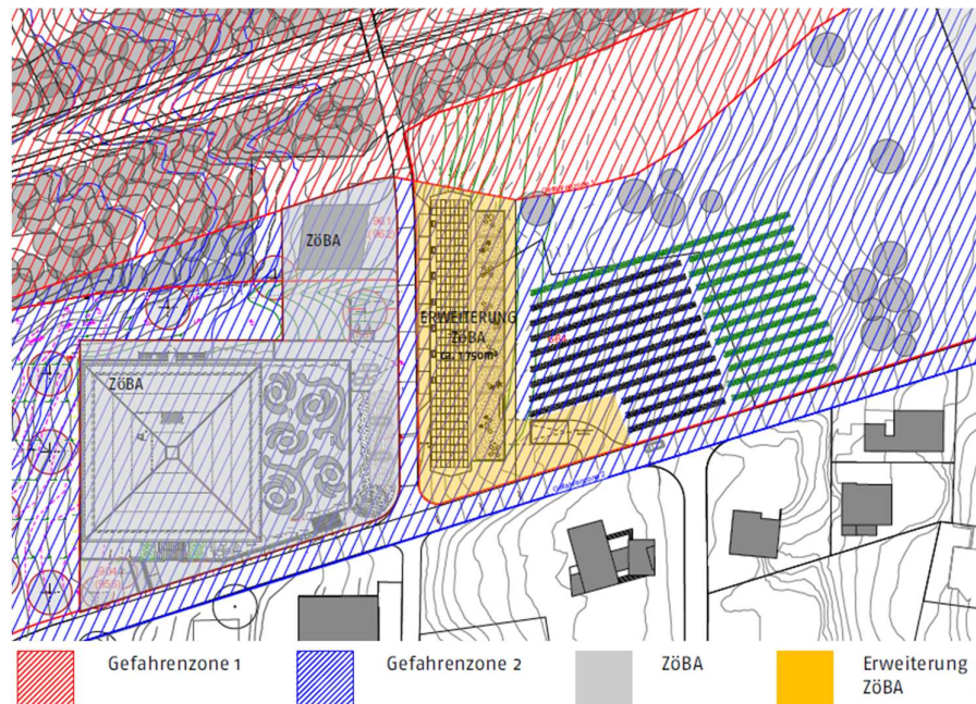
Abb. 5: Situationsplan Studie Neubau Patiententrakt Klinik Gut (Bearth Deplazes Ladner)
