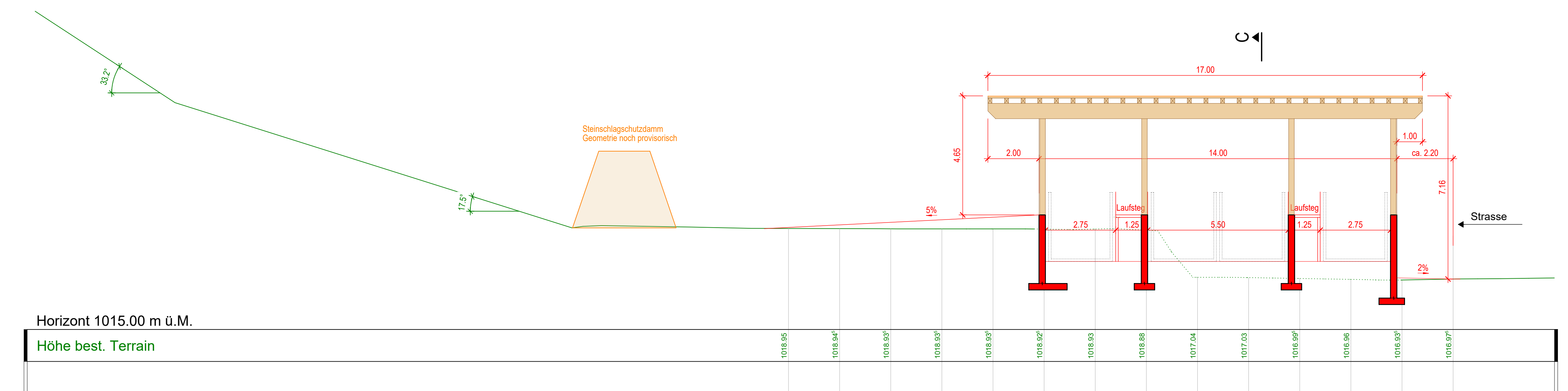
Schnitt B - B 1:100
