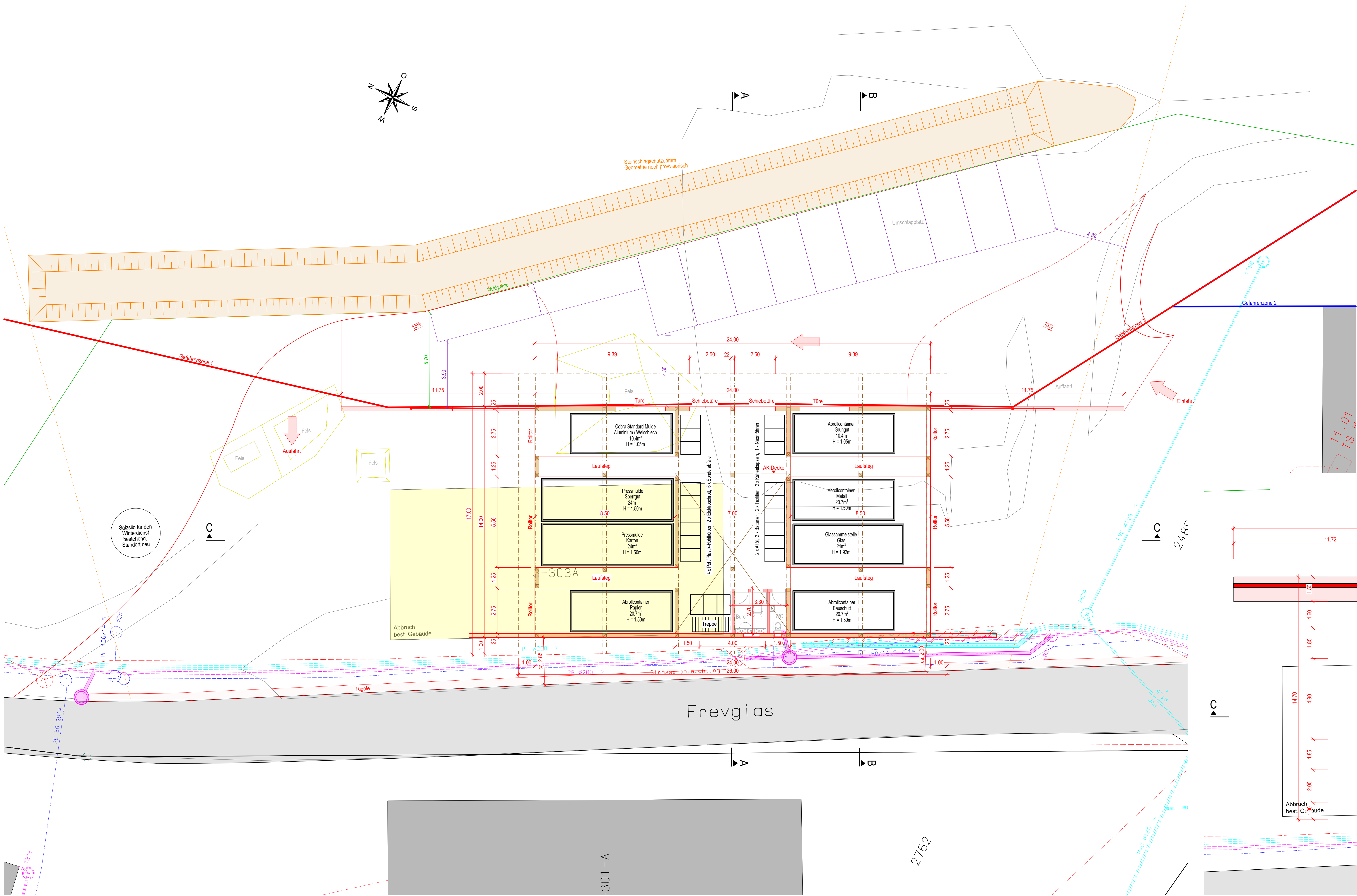
EG Grundriss Draufsicht 1:100
