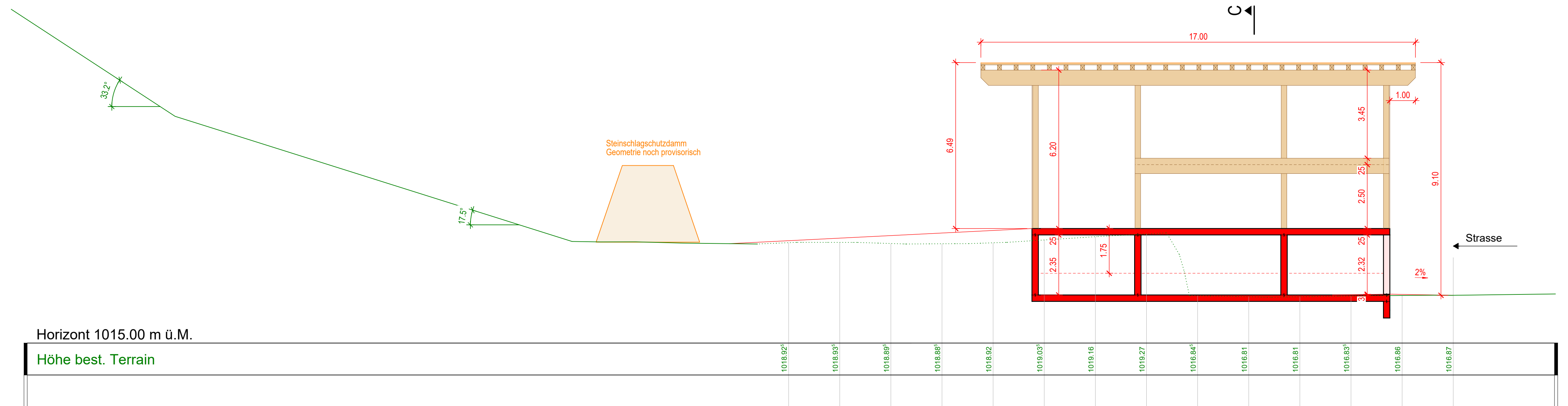
Schnitt B - B 1:100
