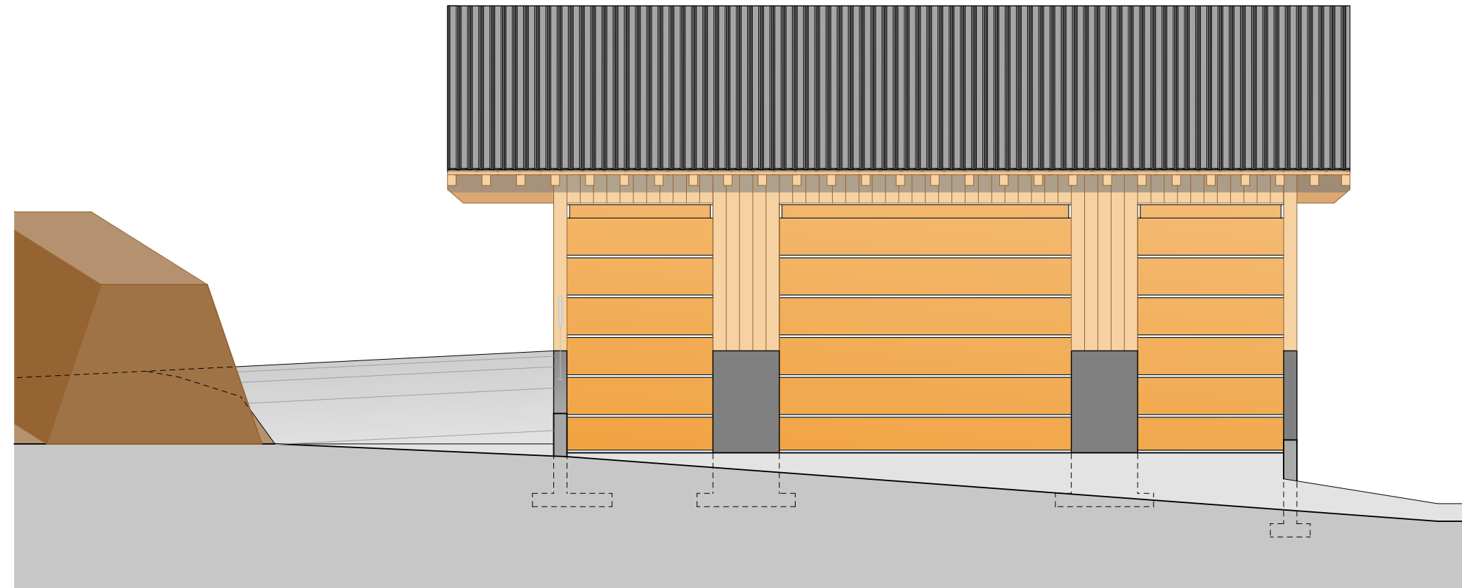
Fassade Nord 1:100
