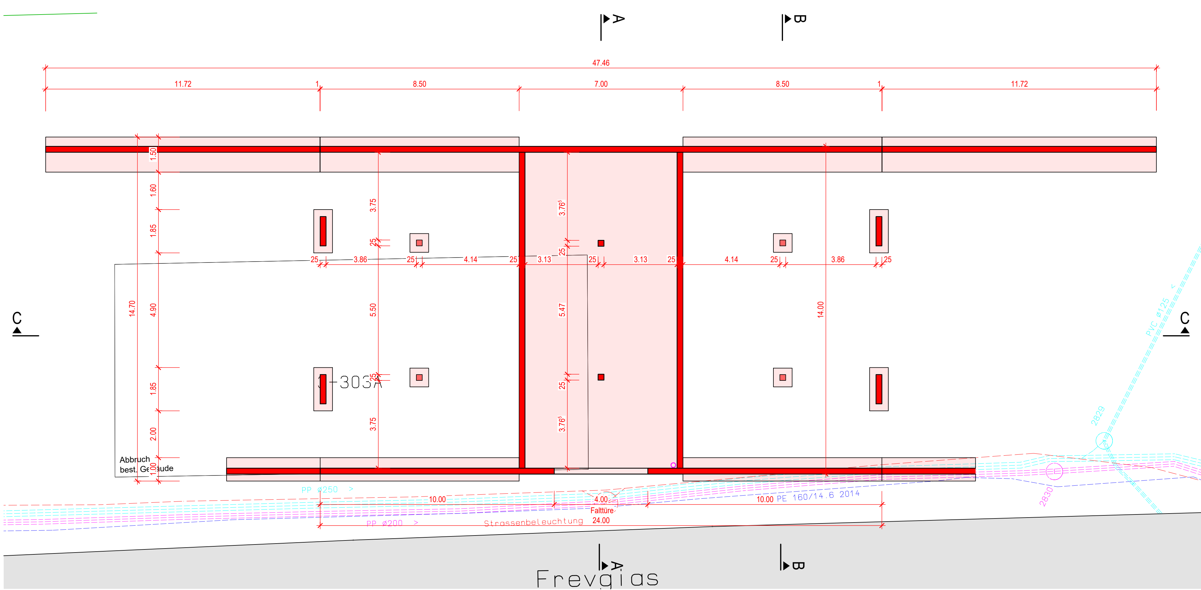
UG Grundriss Draufsicht 1:100
