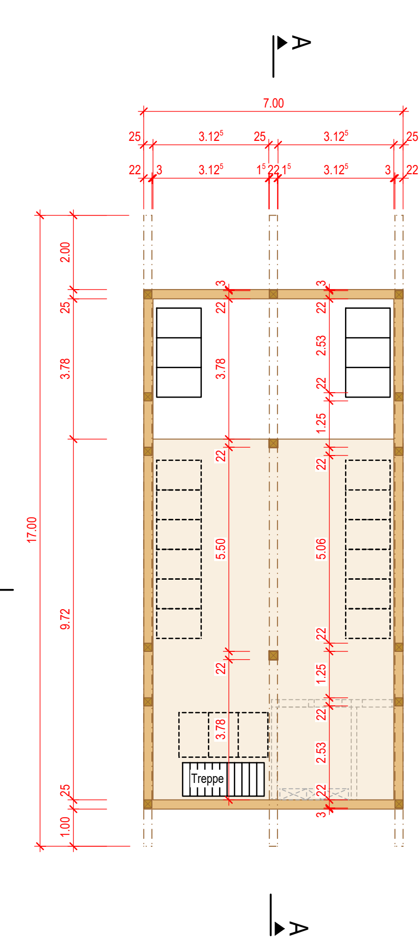
OG Grundriss Draufsicht 1:100
