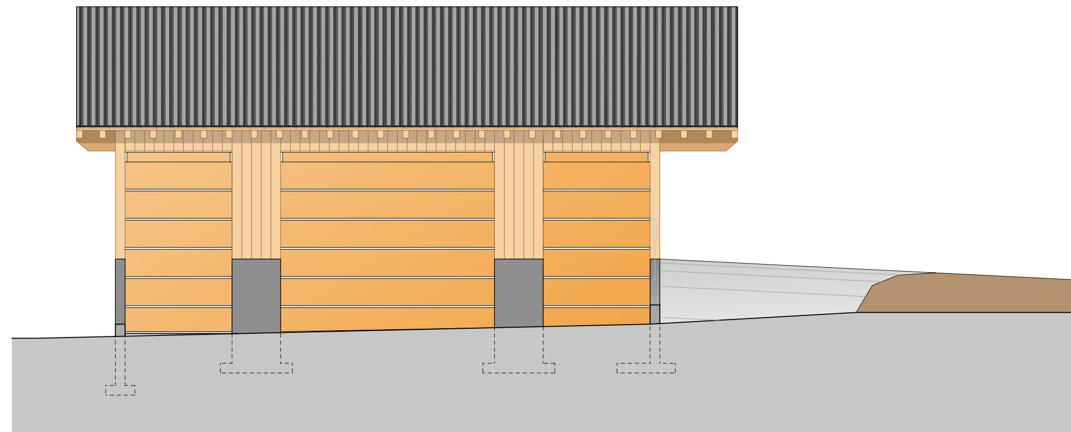
Fassade Süd 1:100
