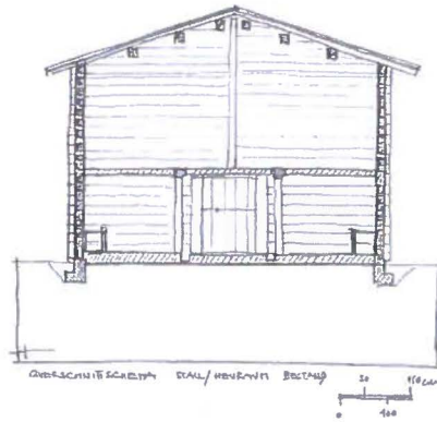
Querschnitt Heukammer/Stallteil
