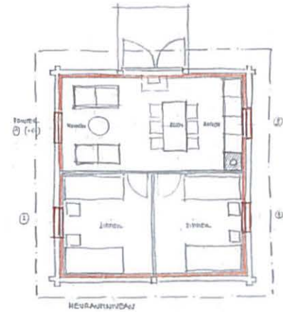
Heuraum mit Wohnräumen und Schlafzimmer
