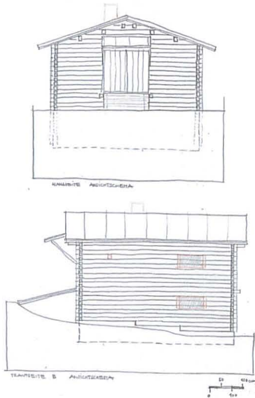
Stallraum zu Wohnzwecken ausgebaut (inkl. Nebenflächen)
