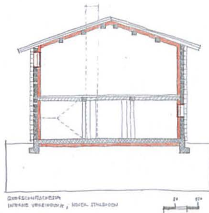
Variante 3 / neuer Stallboden, interne Verbindung
