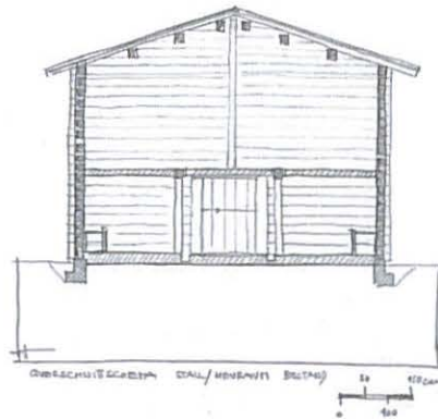
Querschnitt Heukammer/Stallteil
