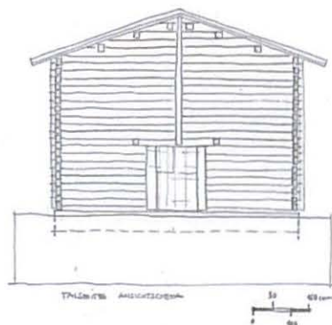
Ansicht talseitig mit Stalltor
