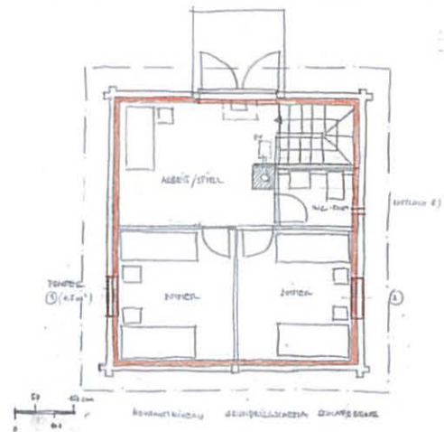
Heuraum mit Schlafräumen und WC ausgebaut,
