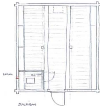
Stallkammer mit WC, Zugang über bestehende Stalltür
