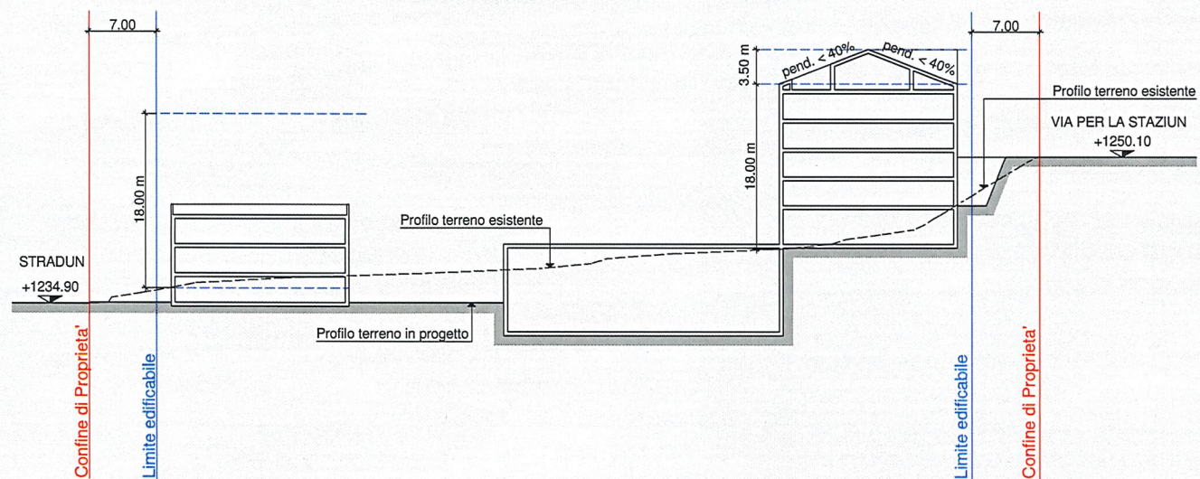
SEZIONE C-C'
