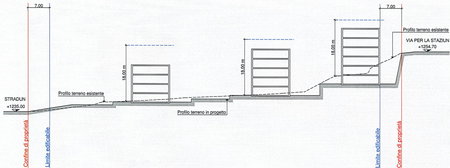
SEZIONE A-A'
