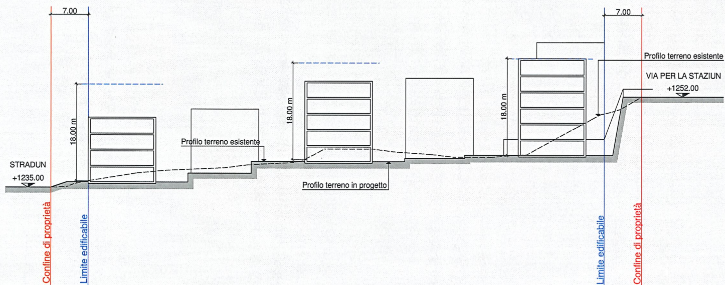
SEZIONE B-B'
