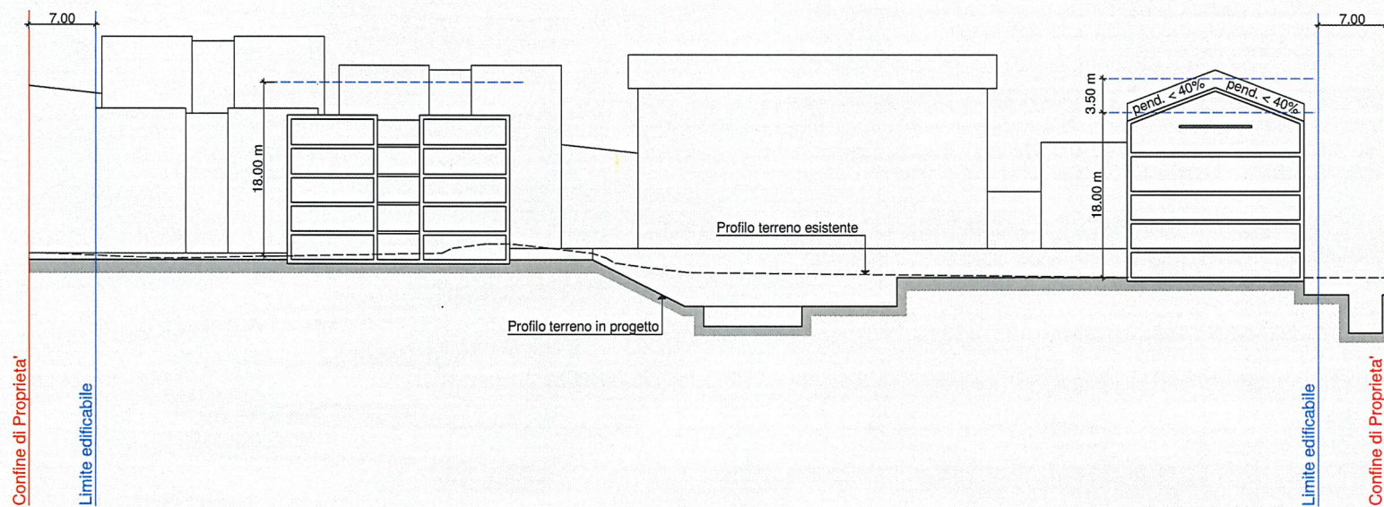
SEZIONE D-D'
