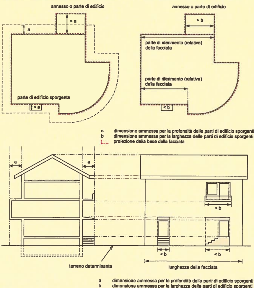
Figure 3.4 Parti di edificio sporgenti (in sezione e in vista laterale)
