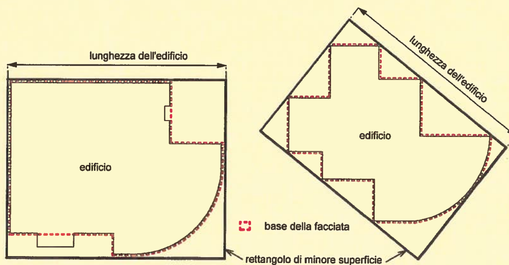
Figura 4.1 Lunghezza dell'edificio
