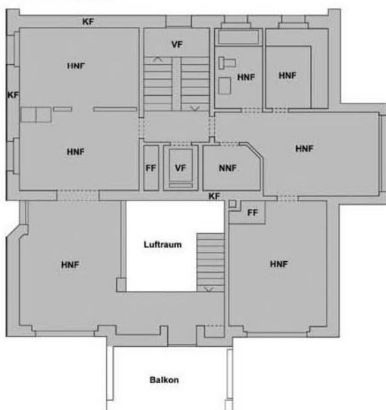
Figur 8.2 Geschossflächenziffer
