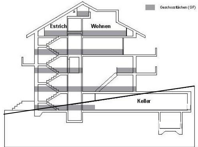
Schnitt:
