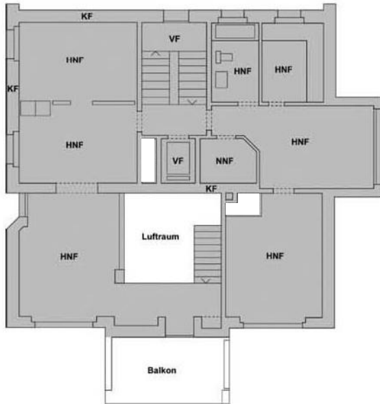
Figur 8.5: anrechenbare Geschossfläche
