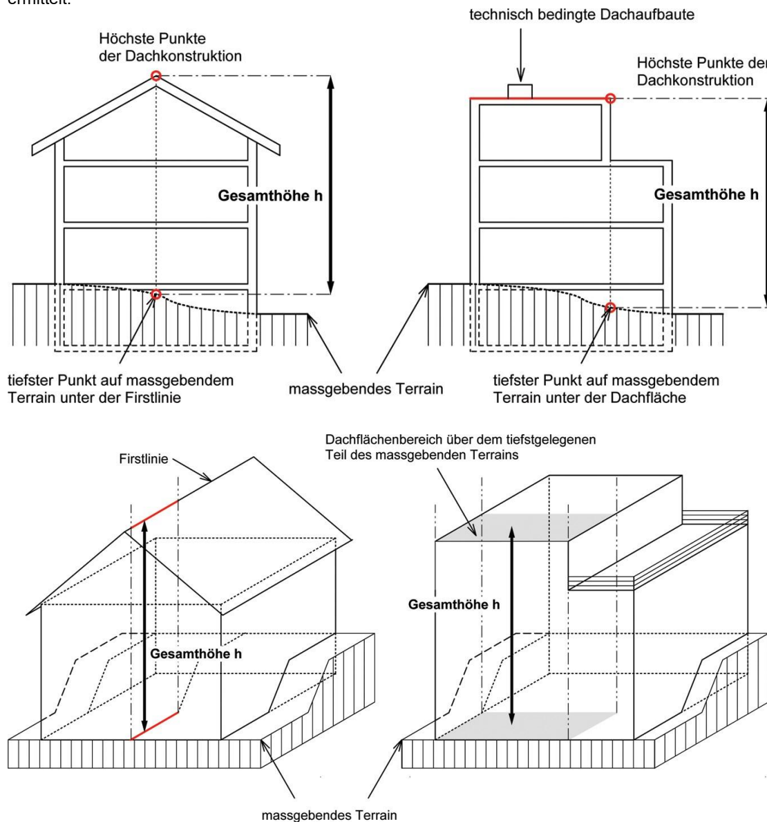
Figur 5.1 Gesamthöhe
