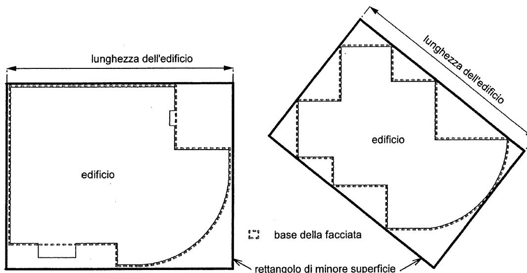
Figura 4.1: Lunghezza dell'edificio
