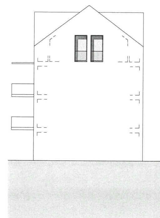
OSTFASSADE
