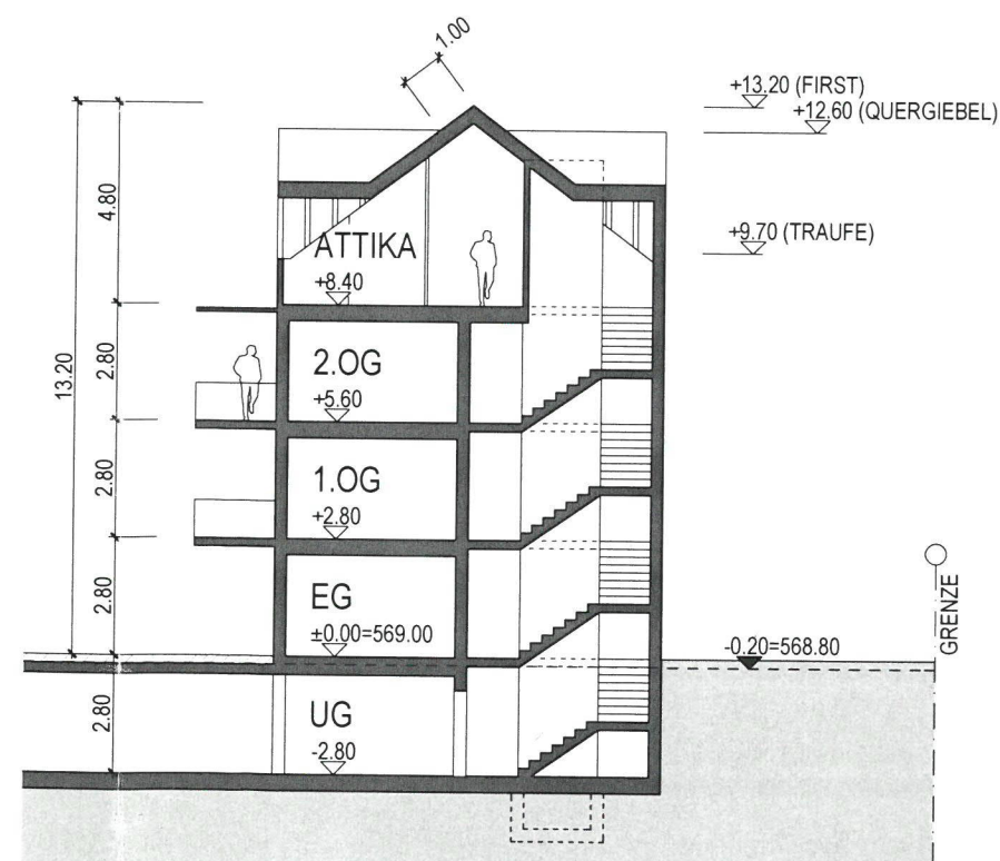
QUERSCHNITT
