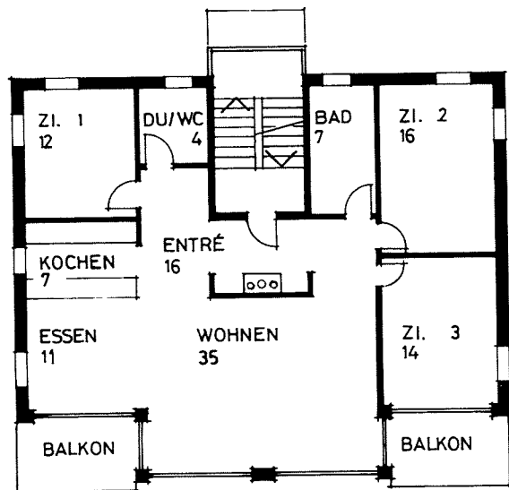
ERDGESCHOSS
