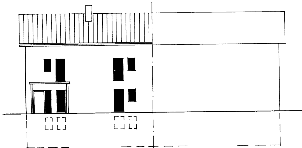
NORDFASSADE
