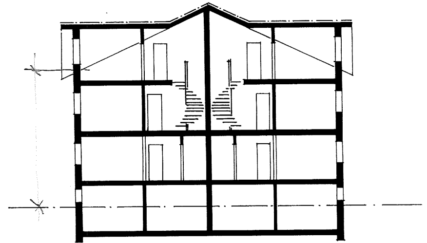
SCHNITT VARIANTE 4
