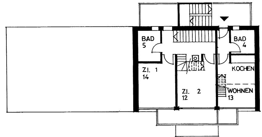
OBERGESCHOSS
