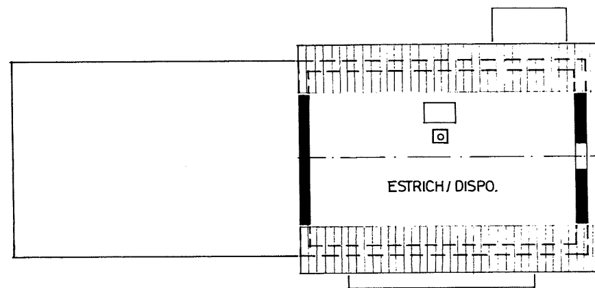
DACHGESCHOSS
