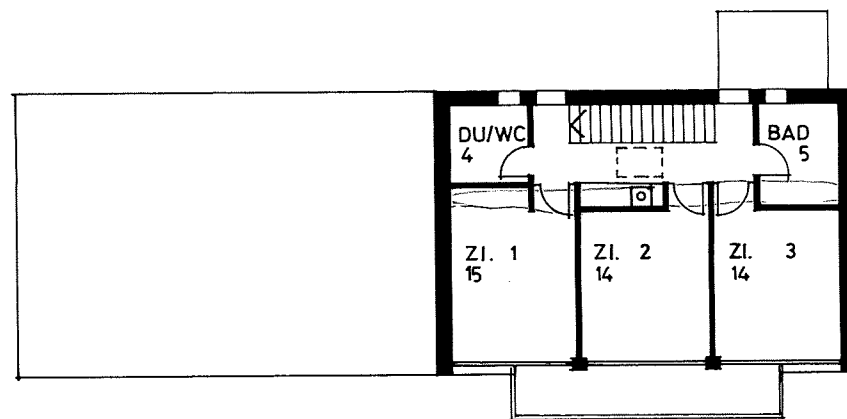
OBERGESCHOSS
