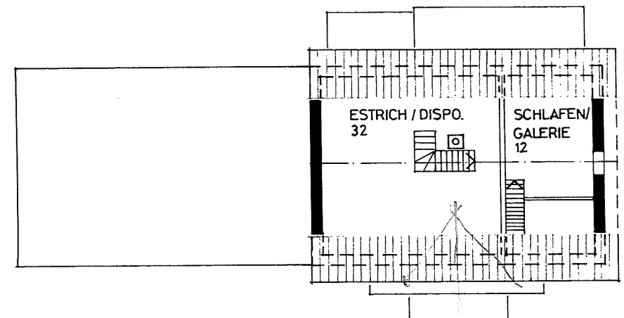
DACHGESCHOSS
