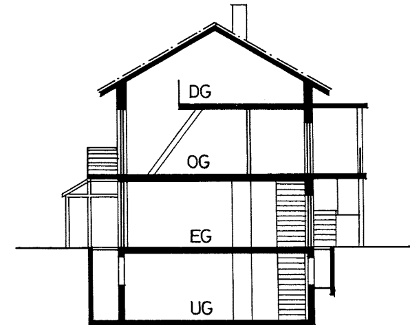
SCHNITT
