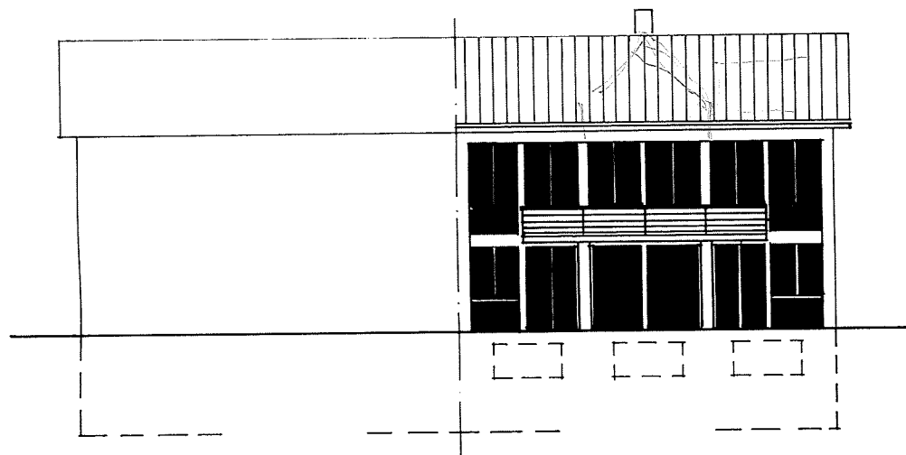
SÜDFASSADE
