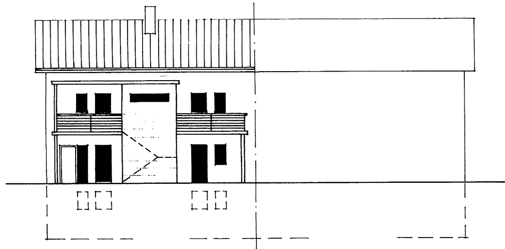
NORDFASSADE
