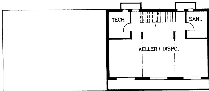
UNTERGESCHOSS
